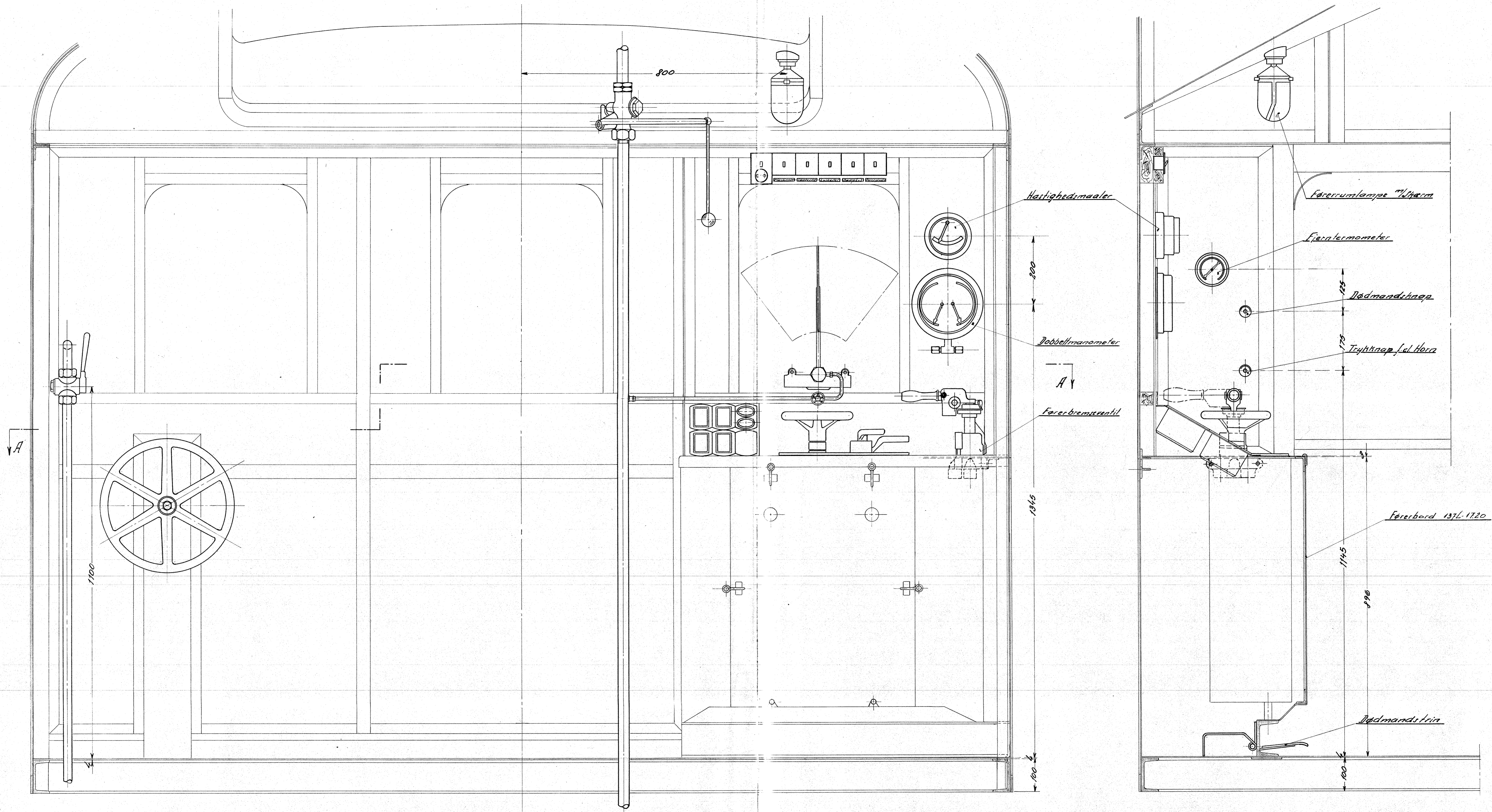
Snit A-A
